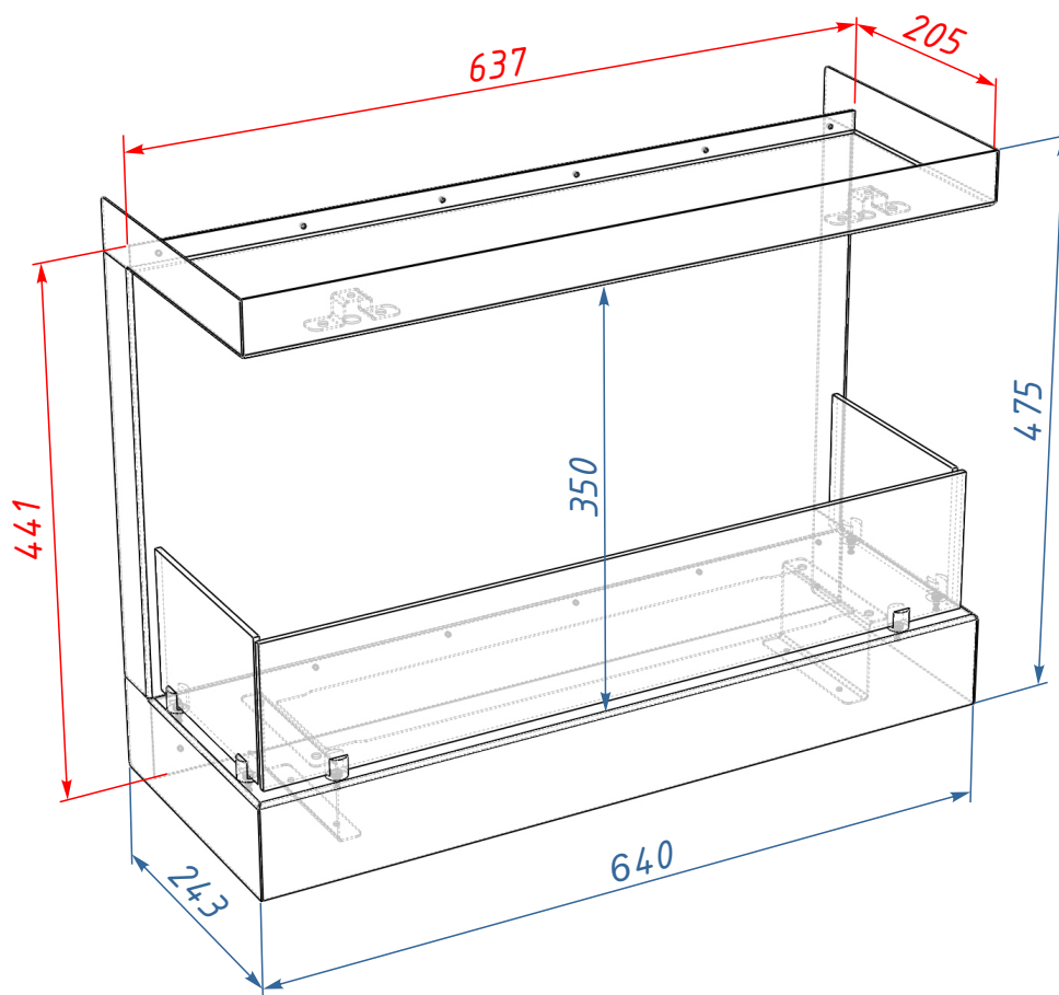
Размеры ниши
