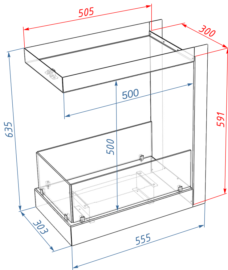
Размеры ниши
