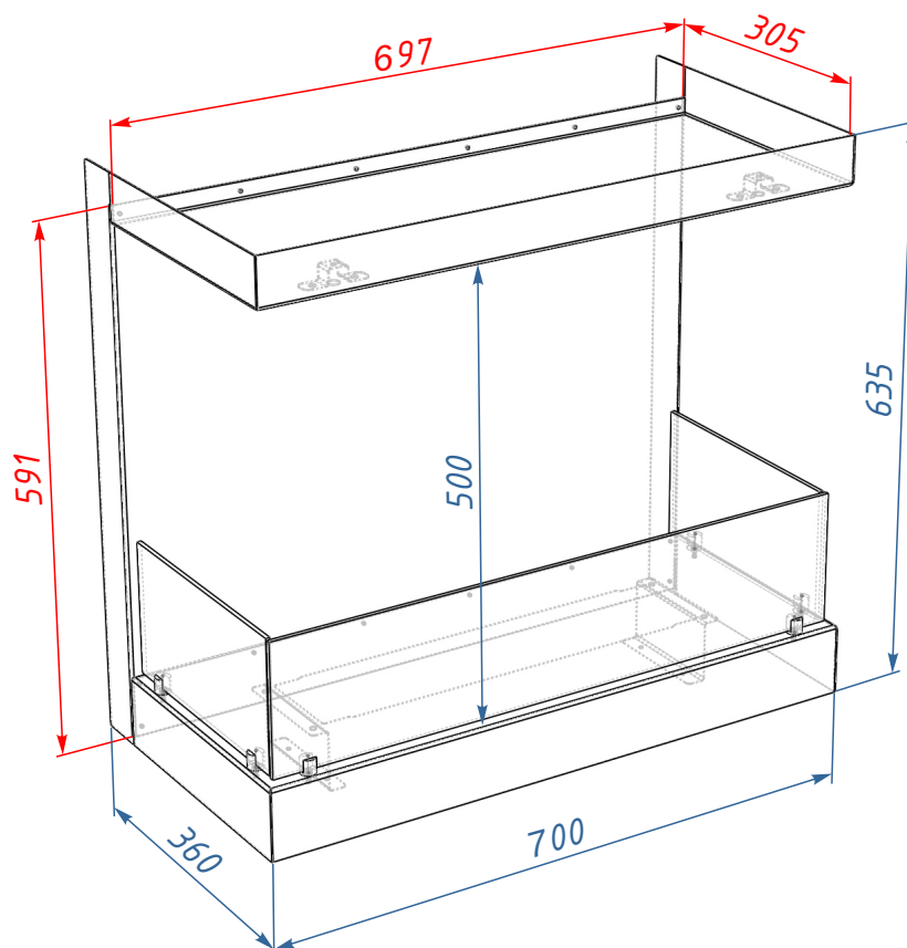
Размеры биокамина
