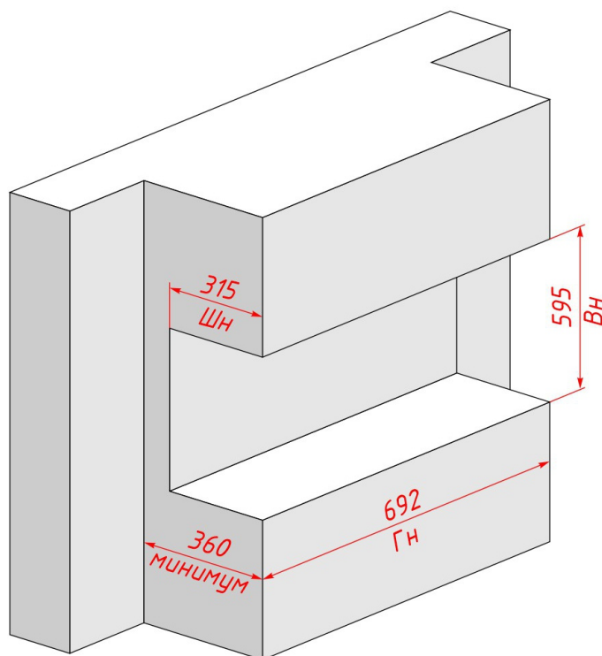
Размеры ниши
