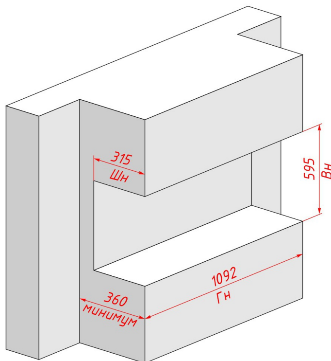
Размеры ниши
