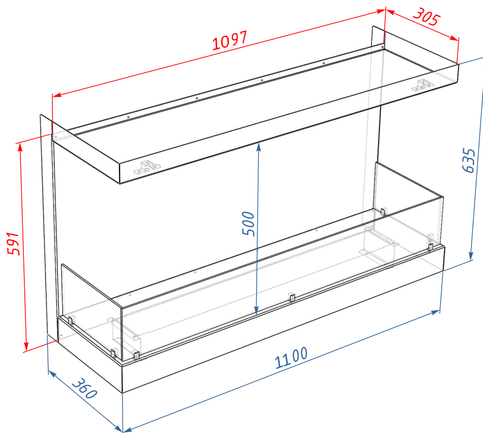
Размеры биокамина
