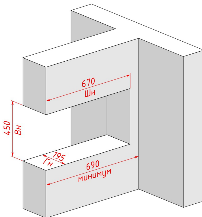
Размеры ниши
