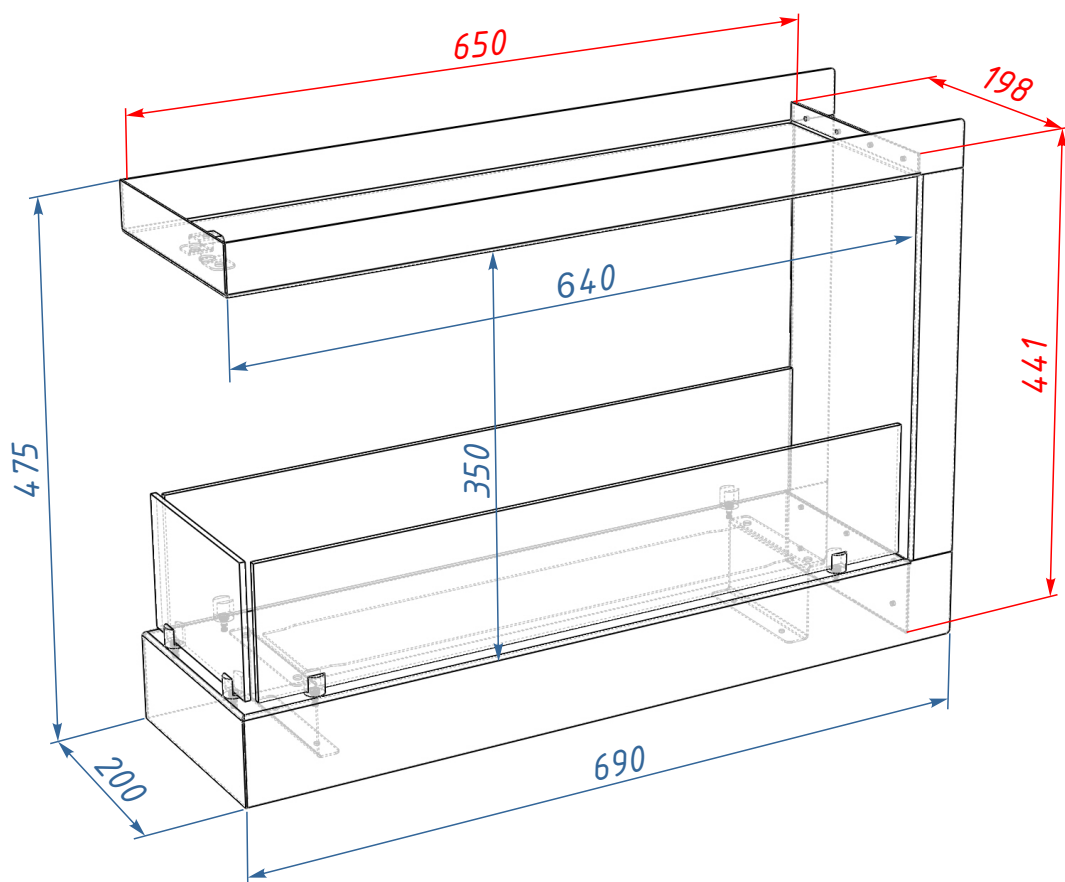
Размеры ниши
